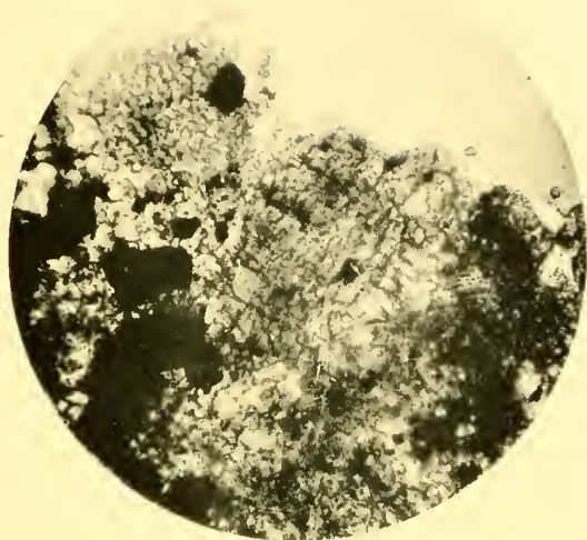
ENSTATITA
