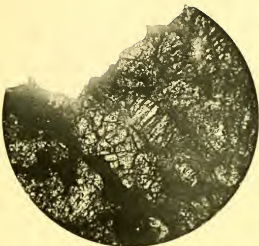
OLIVINO
