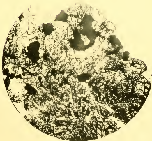
CONDRO OLIVINICO
