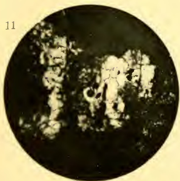
OLIGOCLASA
